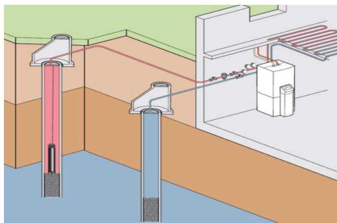
Prinzip-Grundwasserfassung
