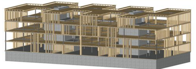
Holzkonstruktion Bitziusstrasse
