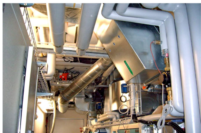
Lüftungszentrale
