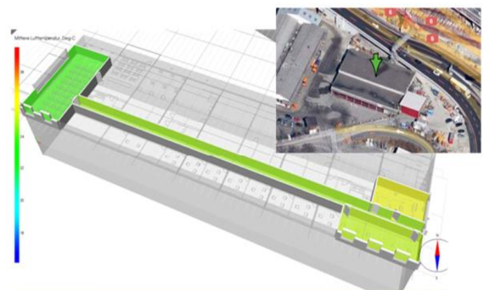
Thermische Simulation
